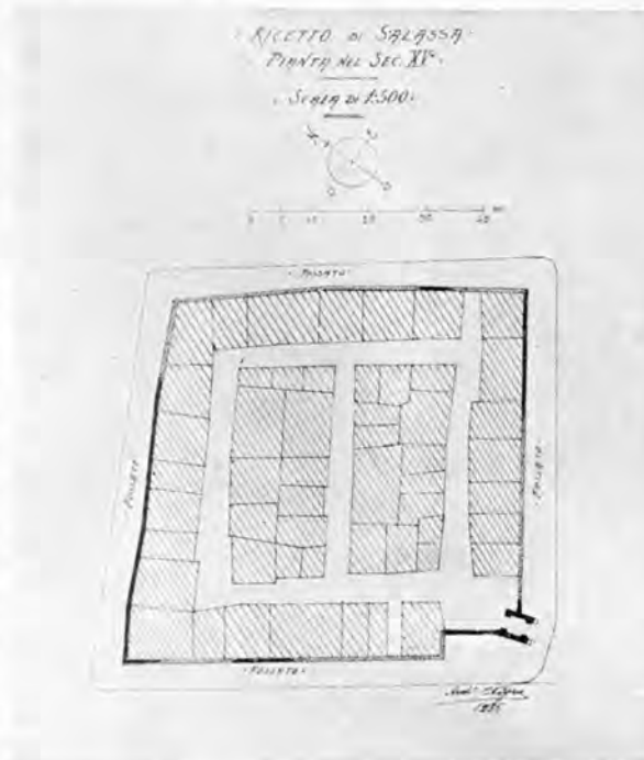
Fig. 13. Ricetto di Salassa - Pianta del sec. XV.
