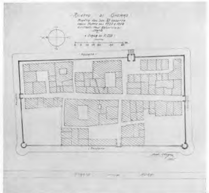
Fig. 34. Ricetto di Ghemme - Pianta del XV secolo.
