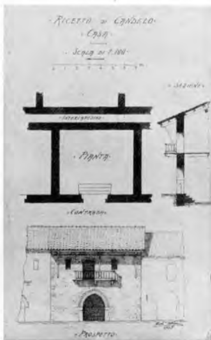
Fig. 26 Ricetto di Candelo - Casa: pianta e prospetto.
