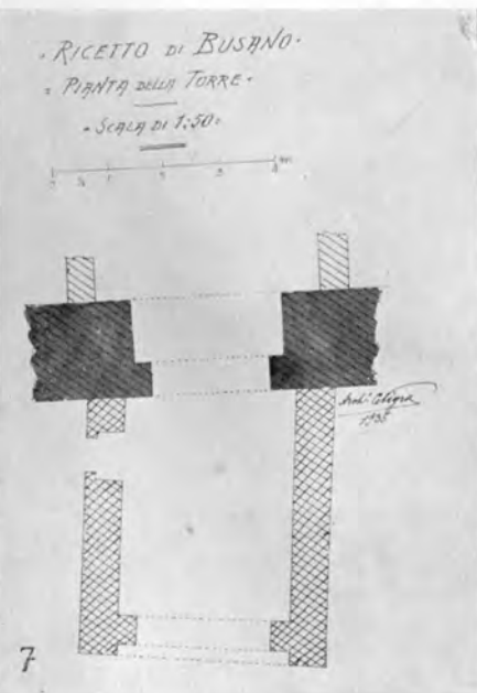
(7) Fig. 11. Ricetto di Busano - Pianta della Torre. — (8) Fig. 19. Ricetto di Candelo - Pianta del XV secolo. — (10) Fig. 21. Ricetto di Candelo - Pianta della Torre.
